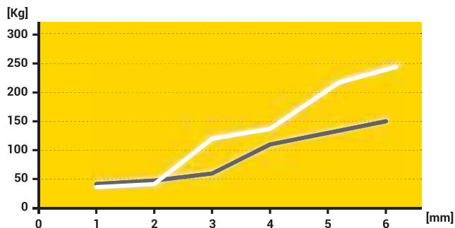
Doporučené ťahové (biela) a šmykové zaťaženie (šedá) v kg a v závislosti na hrúbke plechu vrátane bezpečnostného koeficientu.
