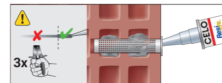
4. Passende Menge Verbundmörtel injizieren (Hülse komplett füllen)
