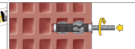
5. Ankerstange drehend eindrücken
