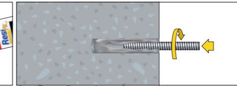
4. Ankerstange drehend eindrücken
